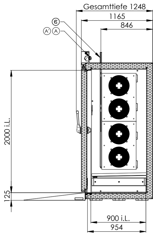
SCHNITT A-A
