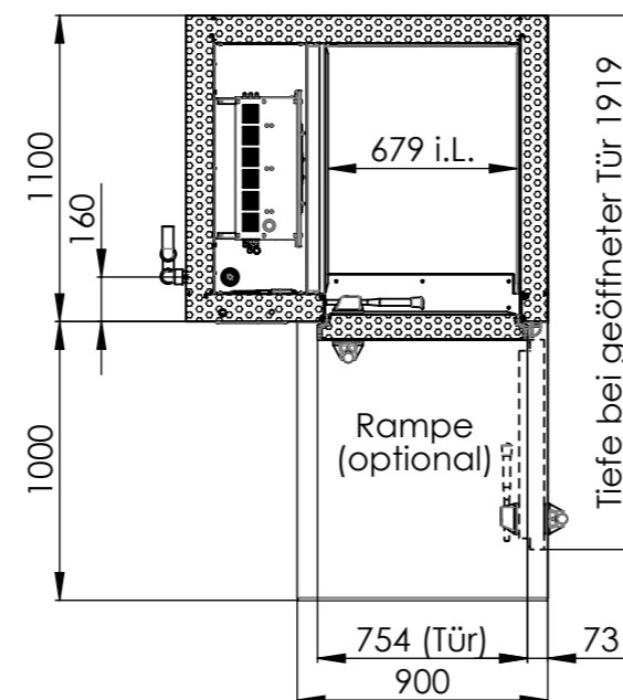
SCHNITT B-B
