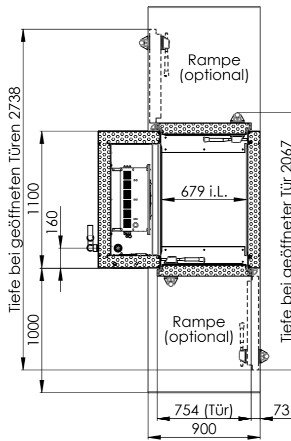
SCHNITT B-B
